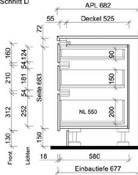
Schnitt D
