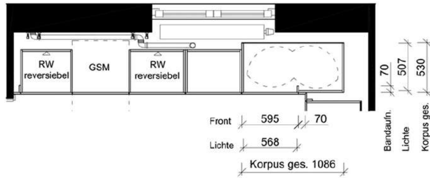
Schnitt C
