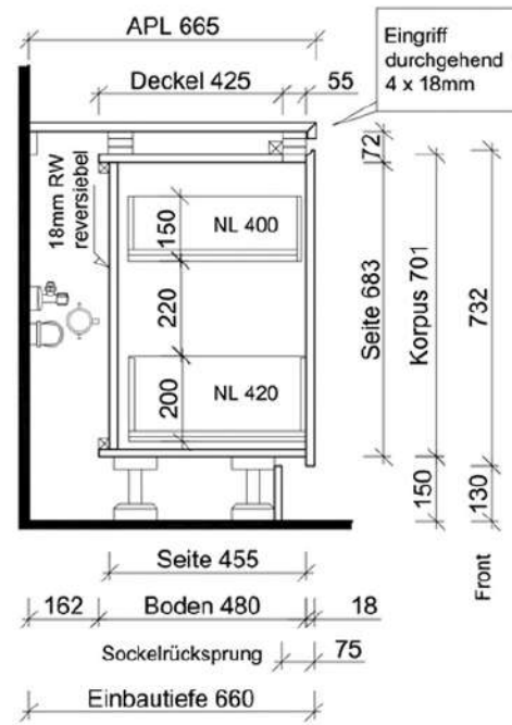
Schnitt D
