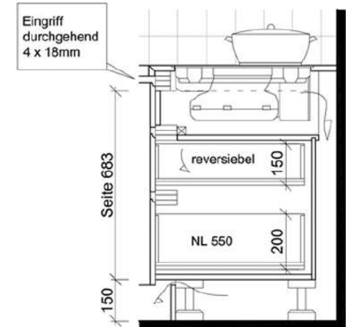
Schnitt E
